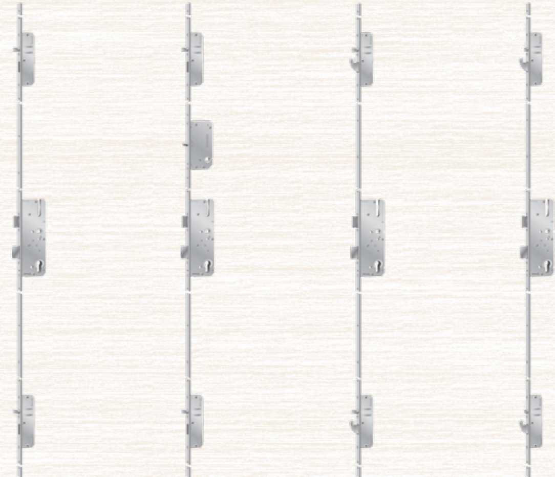
AS 2300 Standardverriegelung Dreifach Bolzenverriegelung
